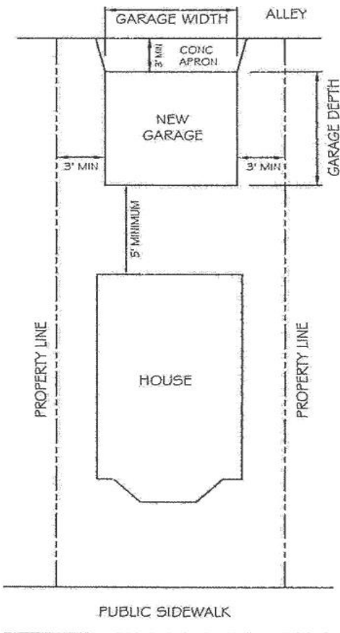
_____ SITE PLAN
